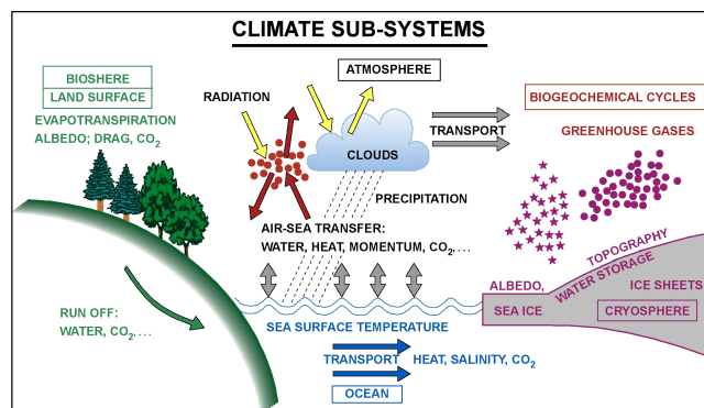
Figur 3. Komponenter af en fuld klimamodel [4].
